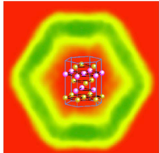
Fermi surface of Bi_2Te_3
